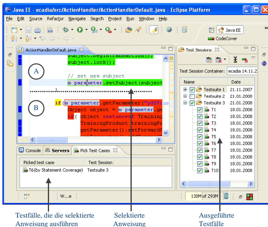
Abbildung 3: CodeCover-Benutzungsschnittstelle
